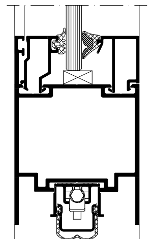
Вертикальное сечение, центрально позиционированное заполнение, масштаб 1:2 Vertical section detail centre glazing, scale 1:2
